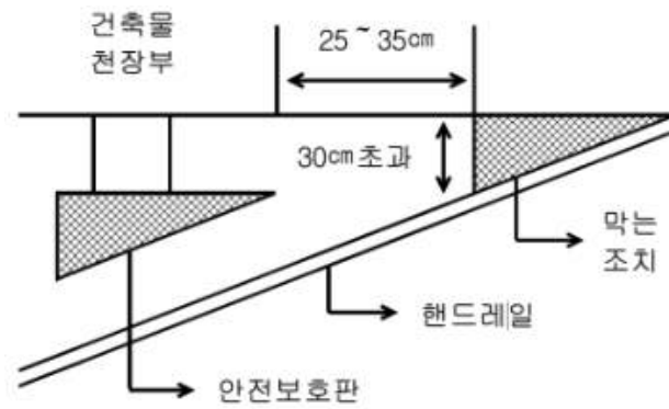
[그림 1.2 - 막는 조치 및 안전 보호판]
