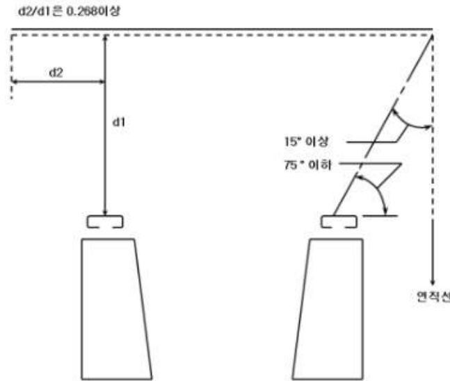
[ 그림 14. 옥외용 에스컬레이터 및 무빙워크의 보호 덮개 ]
