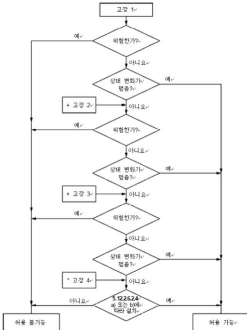
[ 그림 Ⅲ.1 - 고장안전회로의 초안 작성과 평가를 위한 흐름도 ]
