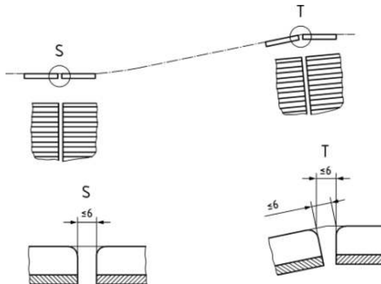
[그림 9 — 팔레트, 상하부 승강장 및 천이구간에서 틈새 및 맞물림 깊이 (맞물리는 홈이 없는 무빙워크의 팔레트 형식)]
