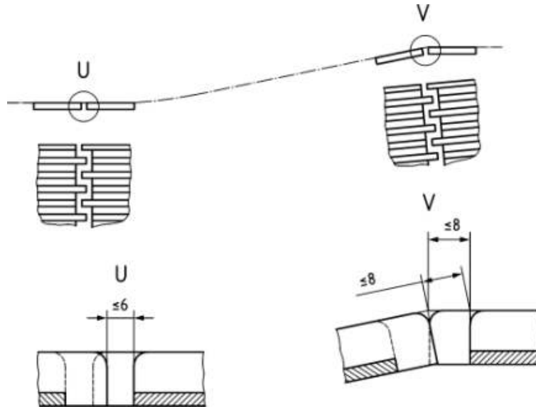
[그림 10 — 팔레트, 상하부 승강장 및 천이구간에서 틈새 및 맞물림 깊이 (맞물리는 홈이 있는 무빙워크의 팔레트 형식)]
