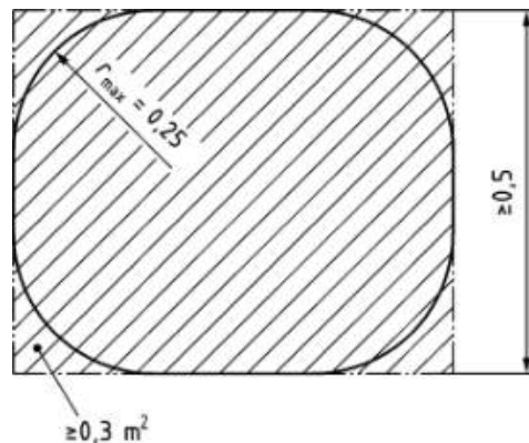
[그림 4 — 서 있을 수 있는 공간]
